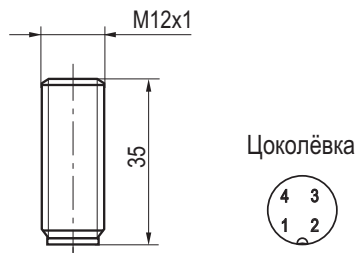
Габаритный чертеж
